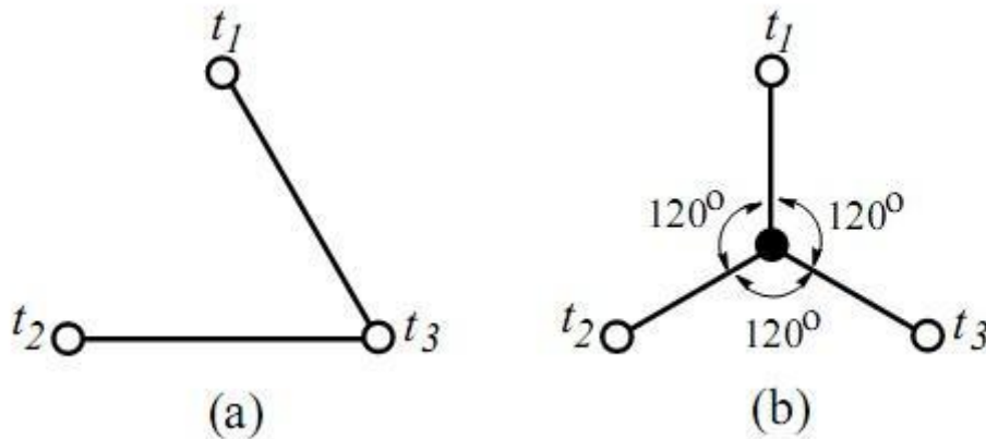
Fig 1. (a) 最小生成树 (b) 斯坦纳树 (来源: Dingzhu Du and Xiaodong Hu [1] )
