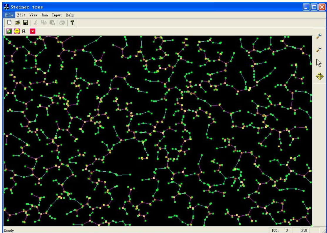
1000 个点的斯坦纳树
