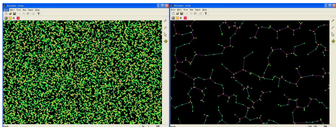
10000 个点的斯坦纳树
