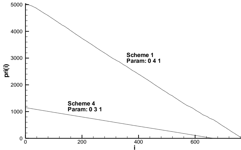
图 5.1 优先级平均差值变化
