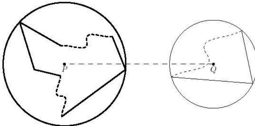
图 4.2 最小包围圆示意
