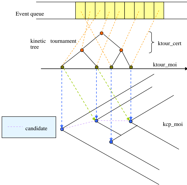
图 13 tournament 结构与 kcp_moi 关系与竞争树结构
