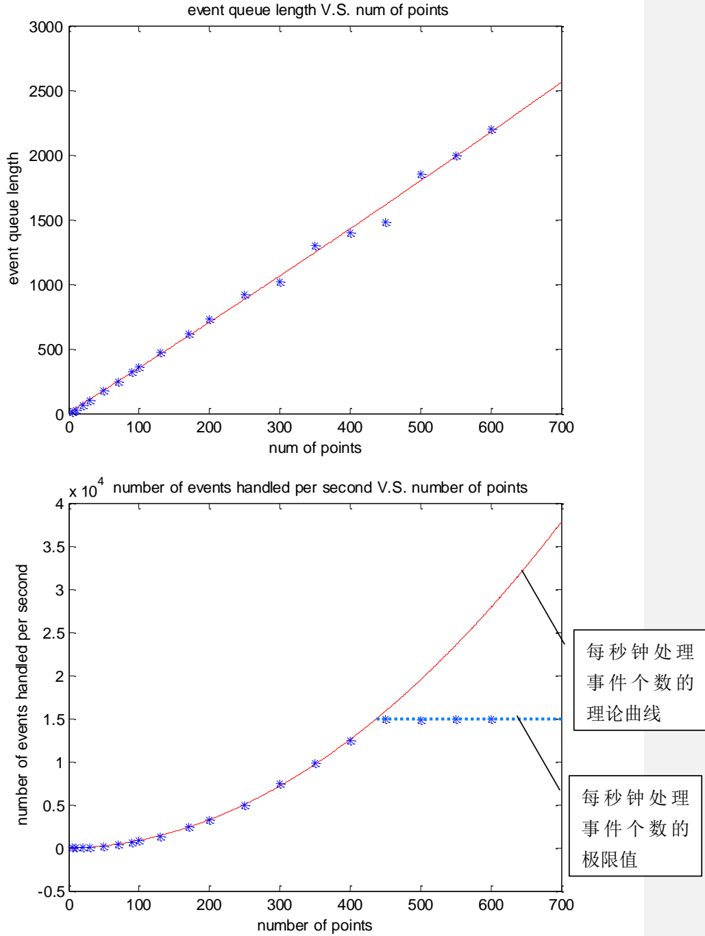
图 15 正常模拟速度下事件队列长度和处理速度与点数关系
