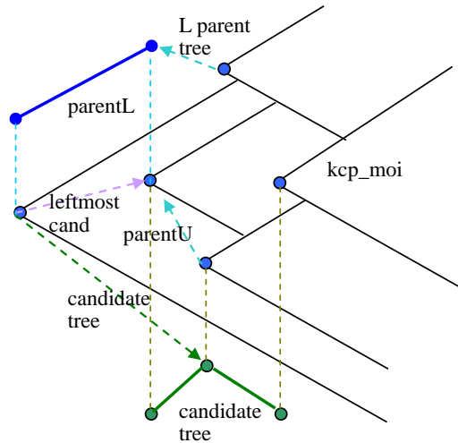
图 10 kcp_moi 主要控制的数据结构关系简图
