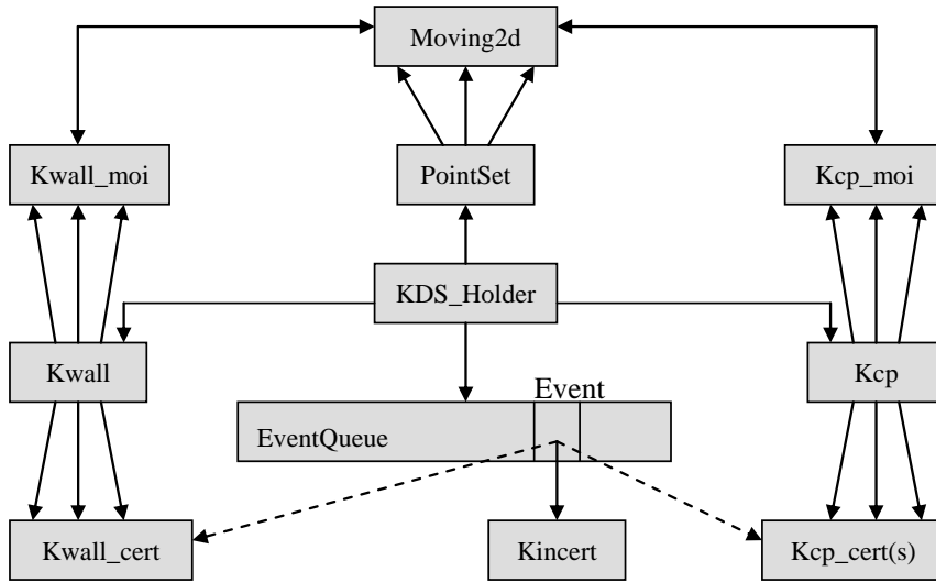
图 7 kds 仿真系统体系结构简图
