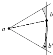
图 2 引理 2 证明
