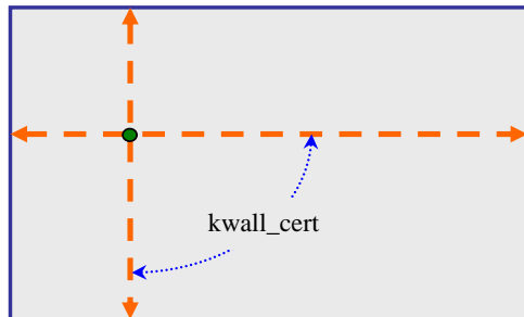
图 14 kwall_cert 示意图
