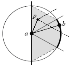
图 1 引理 1 证明
