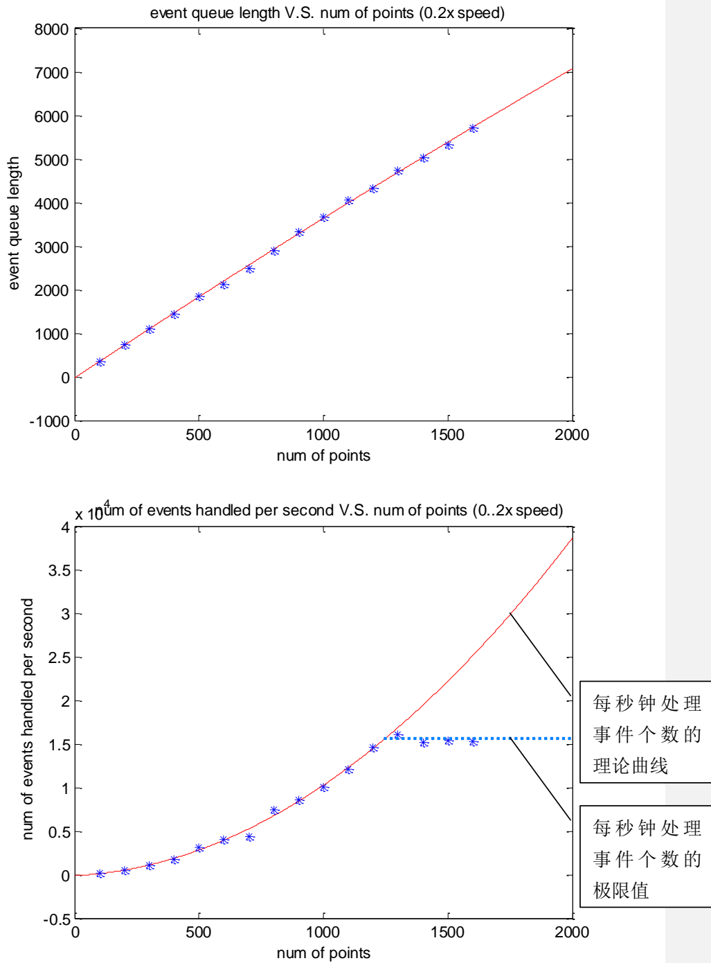
图 16 0.2 倍模拟速度下事件队列长度和处理速度与点数关系
