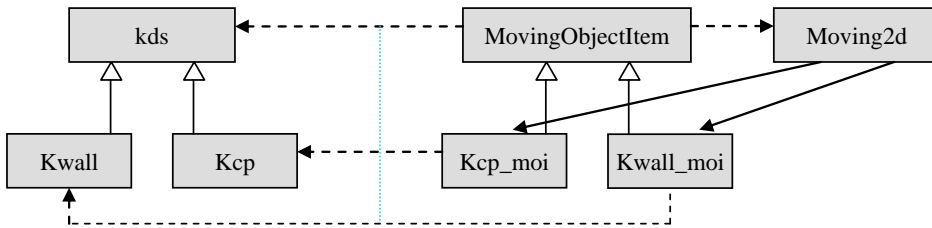
图 8 kcp_moi、kwall_moi 与 kcp、kwall 等的平行继承关系
