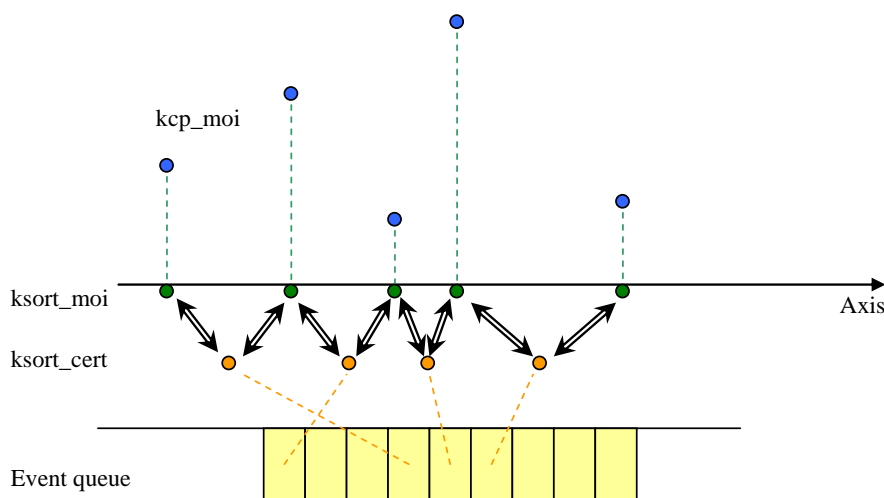
图 11 ksort_cert 与 ksort_moi 关系简图
