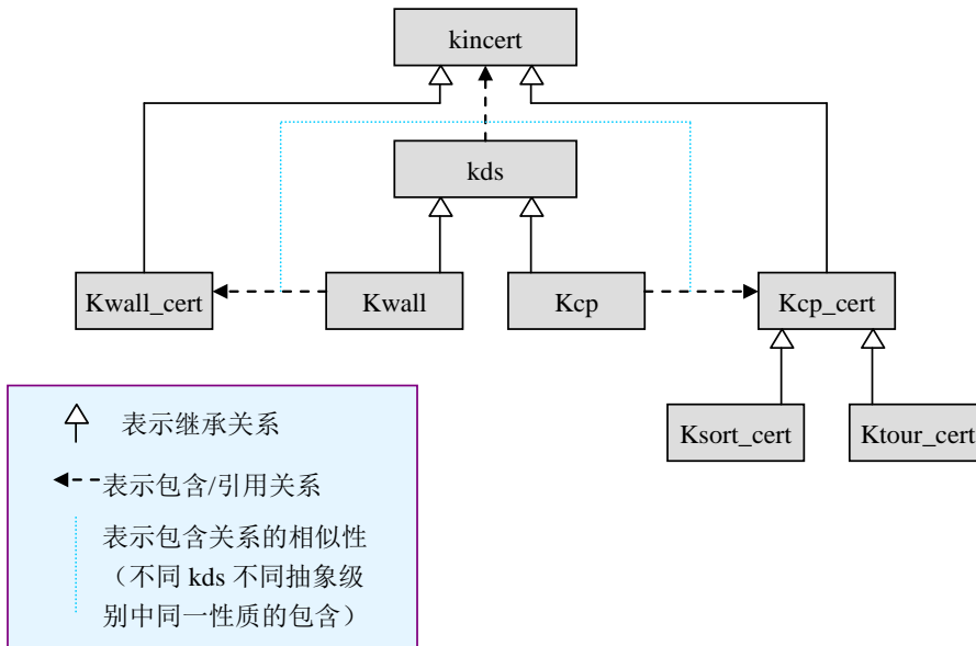
图 9 kcp_cert、kwall_cert 等与 kcp、kwall 等的平行继承关系
