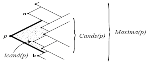
图 3 parent、candidate 等图示
