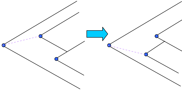
图 12 left candidate 交换示意图
