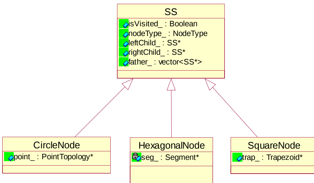
图 5 SS 结构的类之间的继承关系
